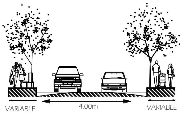
SECCIÓN A-A
