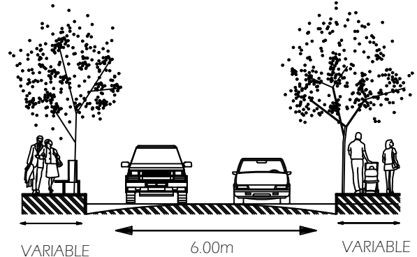
SECCIÓN C-C
